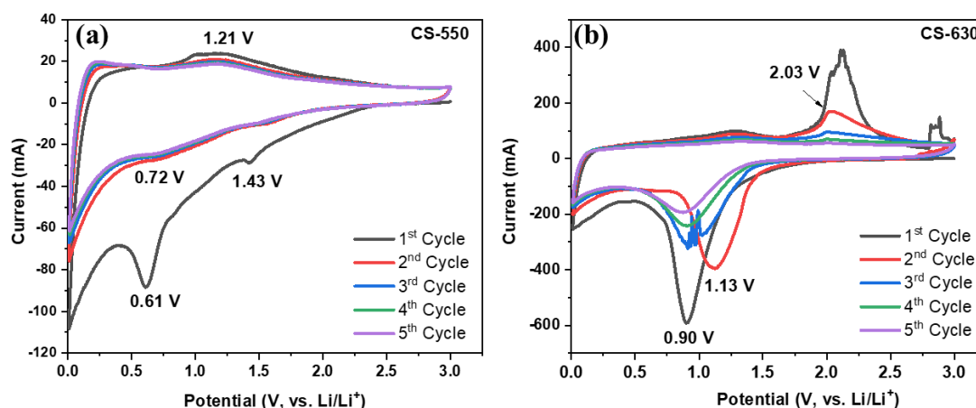
Fig. 3: CV curves of CS-550 and CS-630.
